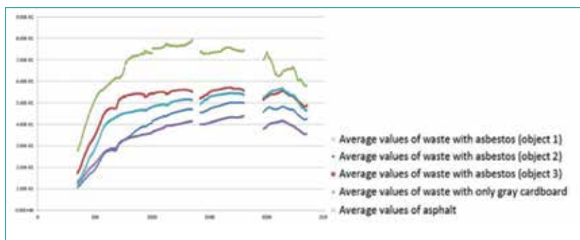
Fig. 10 – Firma spettrale di vari materiali contenenti amianto e dell'asfalto.
